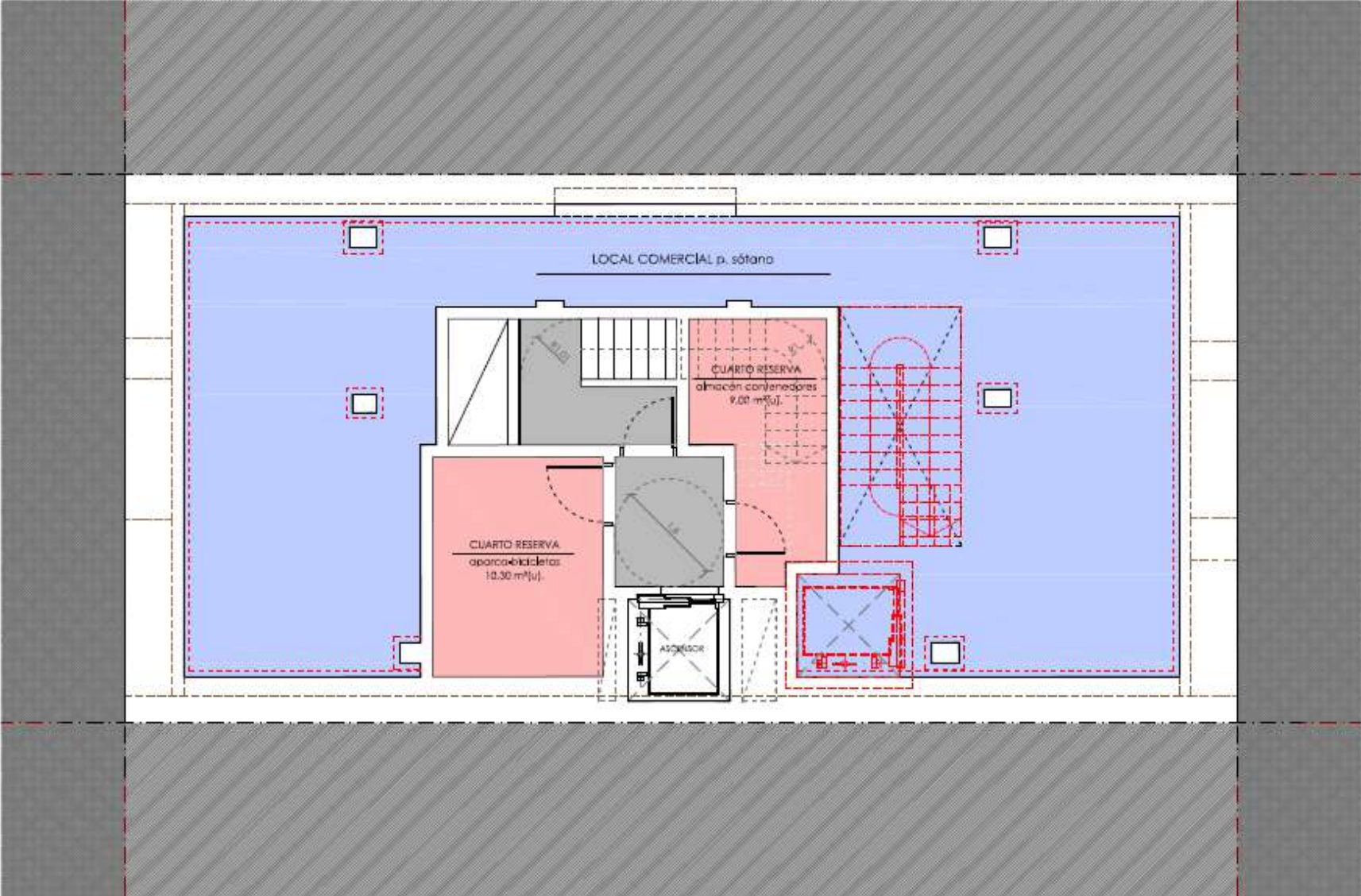
PLANTA SÓTANO
